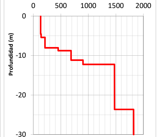
Módulo de Cortante Máxima
