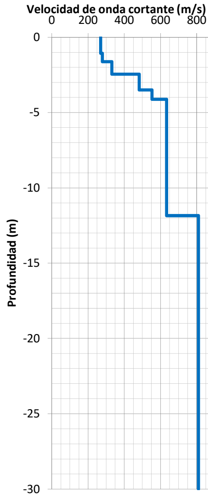
Perfil de velocidad de onda cortante MASW-11
