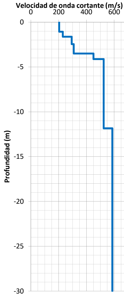
Perfil de velocidad de onda cortante MASW-13
