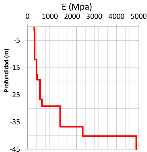
Módulo Elástico
