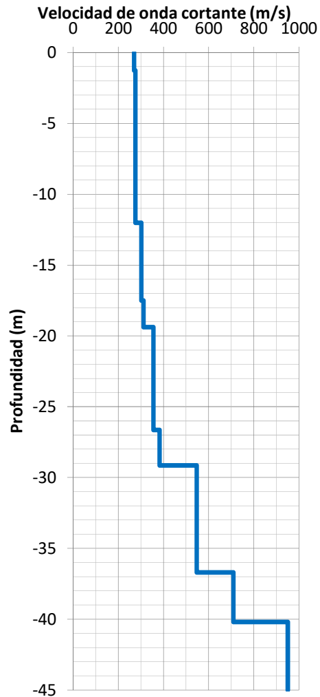
Perfil de velocidad de onda cortante MASW-10
