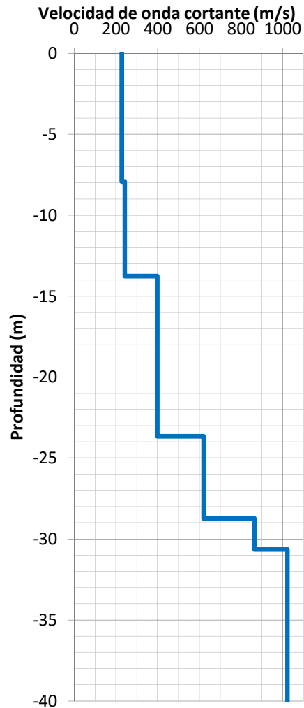
Perfil de velocidad de onda cortante MASW-4
