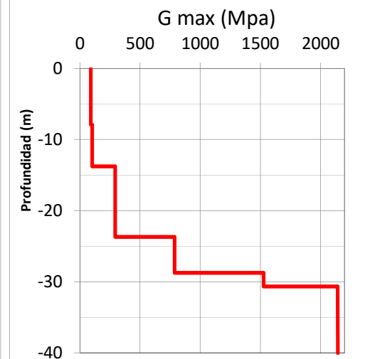
Módulo de Cortante Máxima
