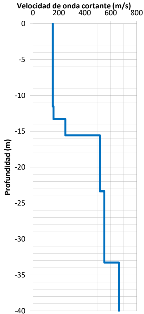
Perfil de velocidad de onda cortante MASW-6
