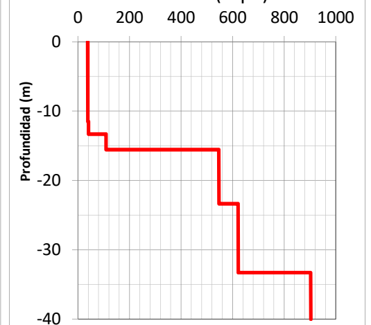
Módulo de Cortante Máxima G max (Mpa)
