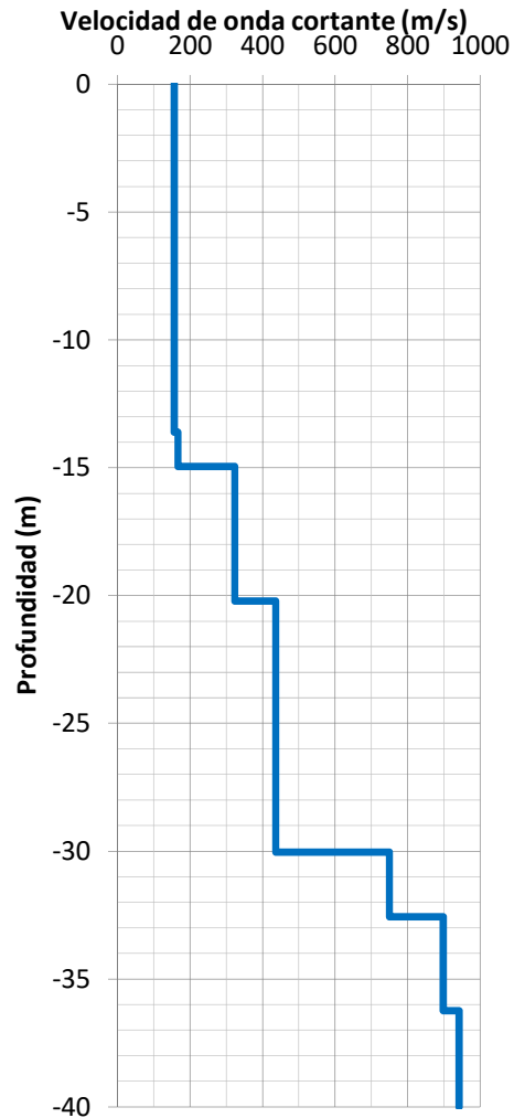
Perfil de velocidad de onda cortante MASW-7
