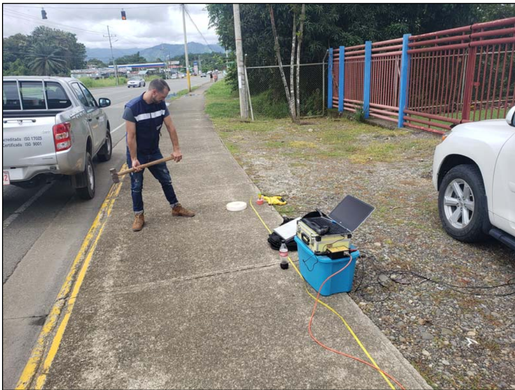
Fotografía 2: Ejecución de ensayo MASW-2
