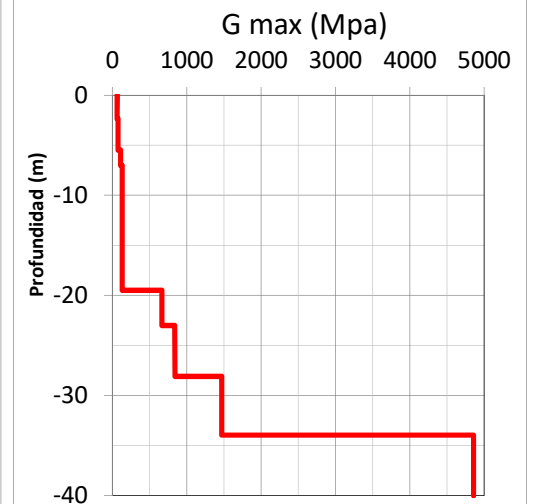
Módulo de Cortante Máxima
