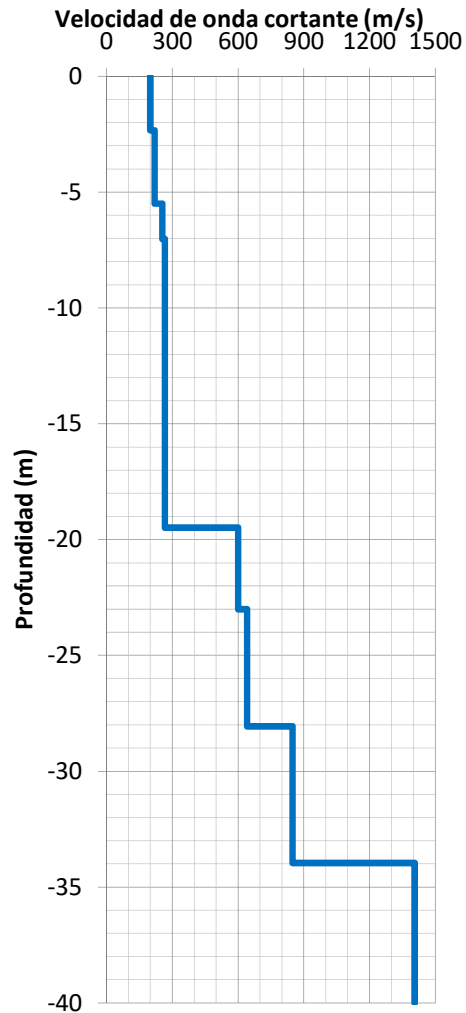
Perfil de velocidad de onda cortante MASW-1
