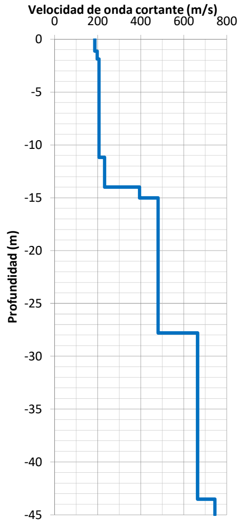
Perfil de velocidad de onda cortante MASW-9
