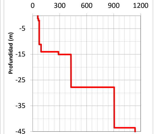
Módulo de Cortante Máxima G max (Mpa)
