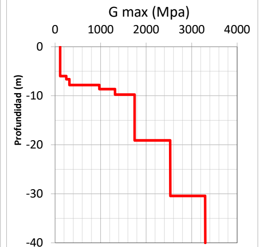
Módulo de Cortante Máxima
