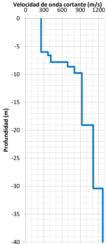
Perfil de velocidad de onda cortante MASW-8
